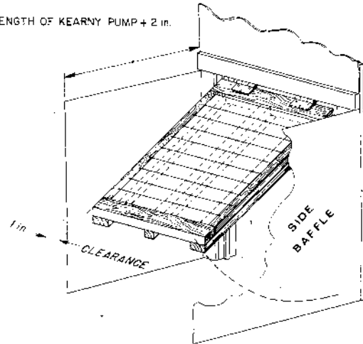
Fig. 25. Side baffles.
